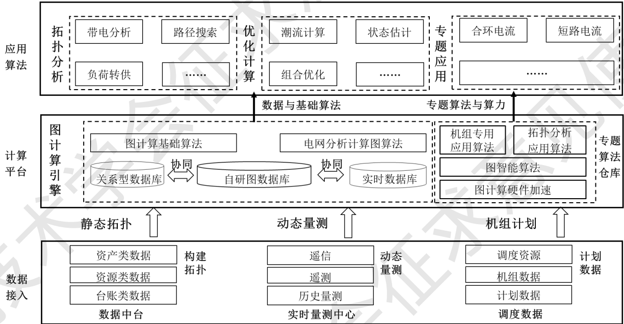
图 1 电力图计算系统参考架构
